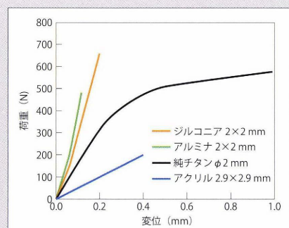
図1 3点曲げ試験時の荷重-変位曲線(文献 1) より引用・改変)。
