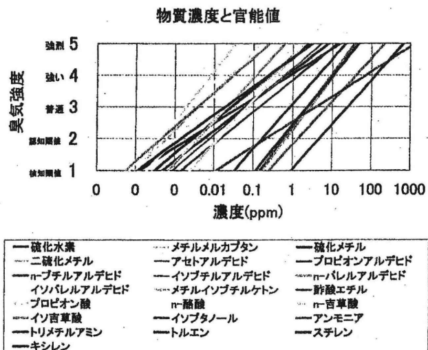
図 2 物質濃度とにおいの強さの関係
