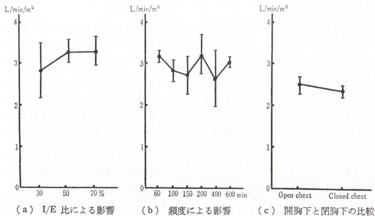
図 7 左右肺独立換気時の CI の変化 (mean ± SEM)
