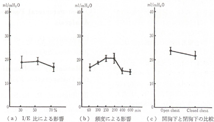
図 5 左右肺独立換気時の C dyn の変化 (mean ± SEM)
